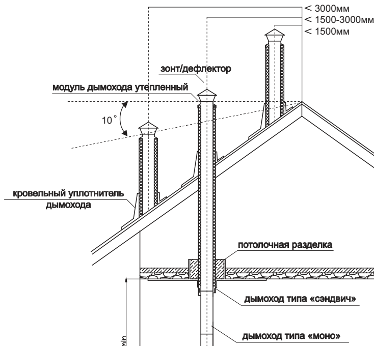
Рис.9 Возвышение дымовых труб над кровлей (согласно СНиП-91 п.3.73.)
